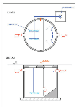
Schema di depuratore con vasca a pianta circolare
