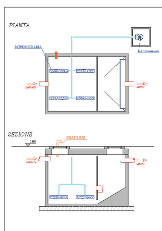
Schema di depuratore con vasca a pianta rettangolare
